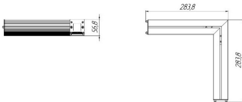
Рисунок 5 Светильник «L-fusion Retail MG L»
